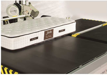
Faultless synchronization system sewing machine and conveyor belt. Dikiş makinasının ve konveyer bandının mükemmel uyumu
